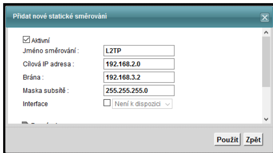
Obrázek 13-6 Příklad konfigurace L2TP VPN tunelu na 3. vrstvě, Přidat nové statické směrování
