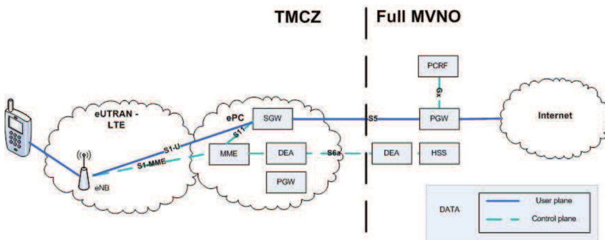
obr. 1: Technické řešení
