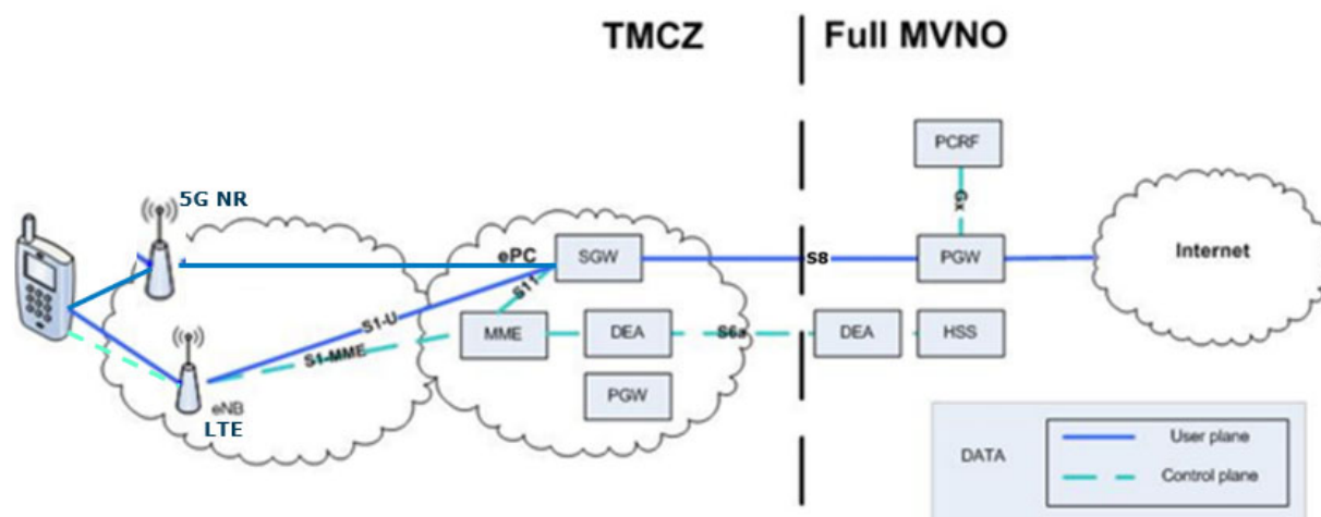
obr. 1: Technické řešení
